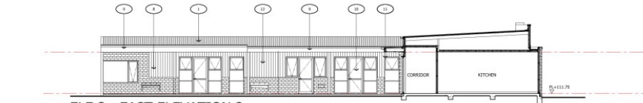
ELE 3 - EAST ELEVATION 2 SCALE 1:100
